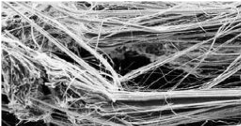
Rasterelektronenmikroskopische Aufnahme von Asbestfasern
